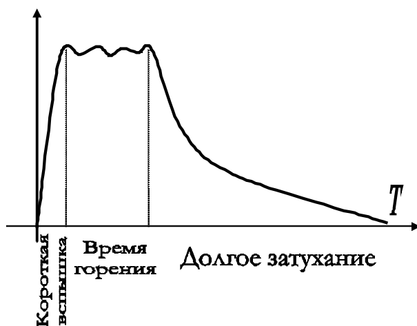
Рис. 5. График функции «взрыва порохового склада»
